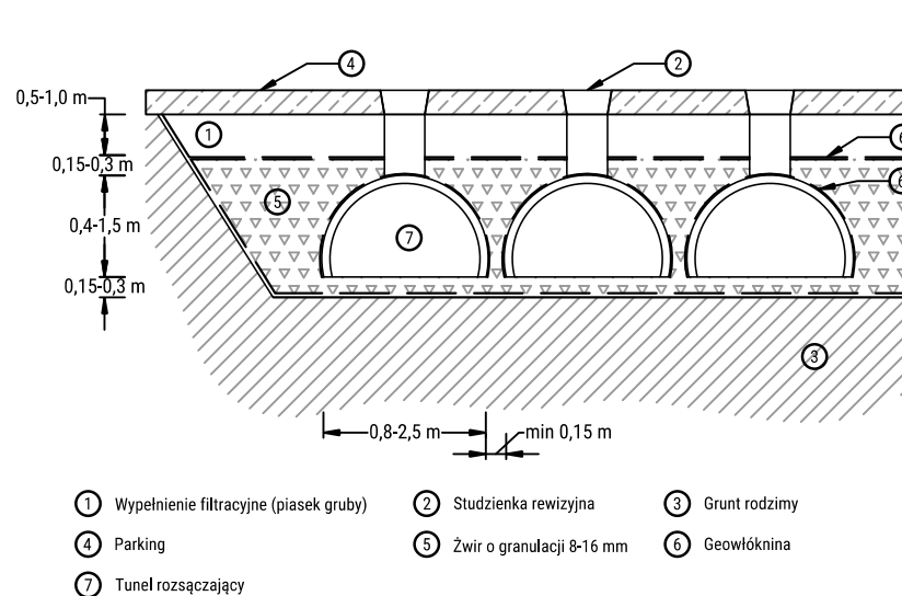
Przekrój poprzeczny przez instalację składającą się z kilku komór drenażowych
