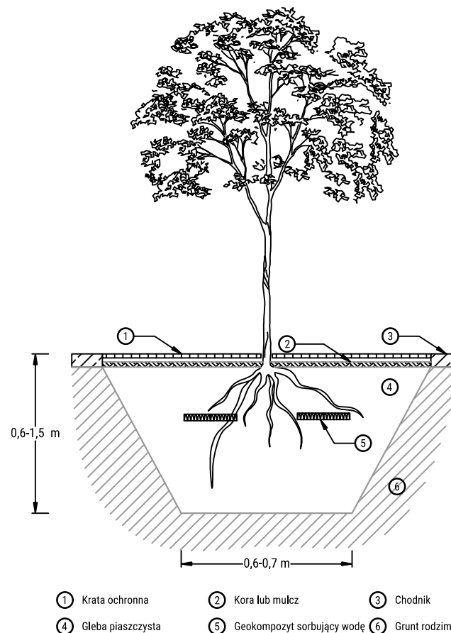
GSW wykorzystane w nasadzeniach drzew
