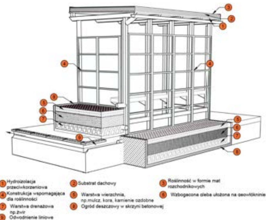
Schemat zielonego przystanku
