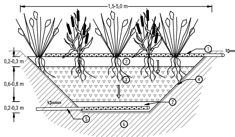
Przykład obiektu hydrofitowego z przepływem poziomym
