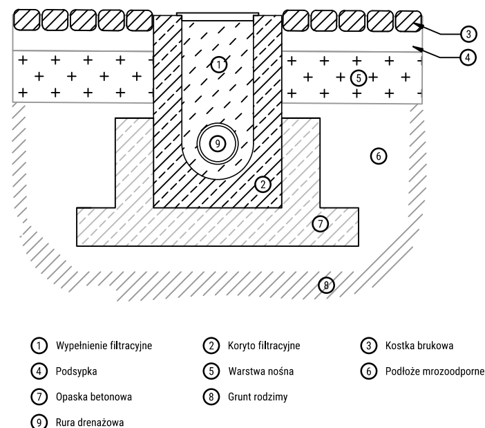
Korytko filtracyjne
