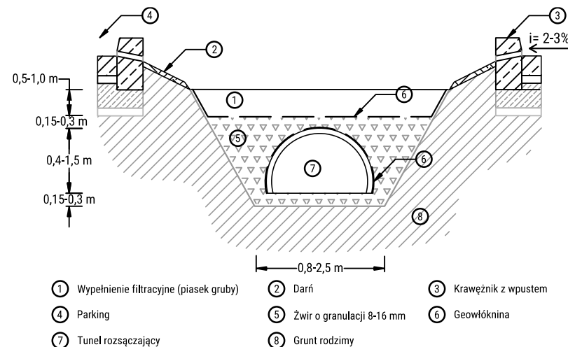
Przekrój przez rów odwadniający z zastosowaniem komór drenażowych
