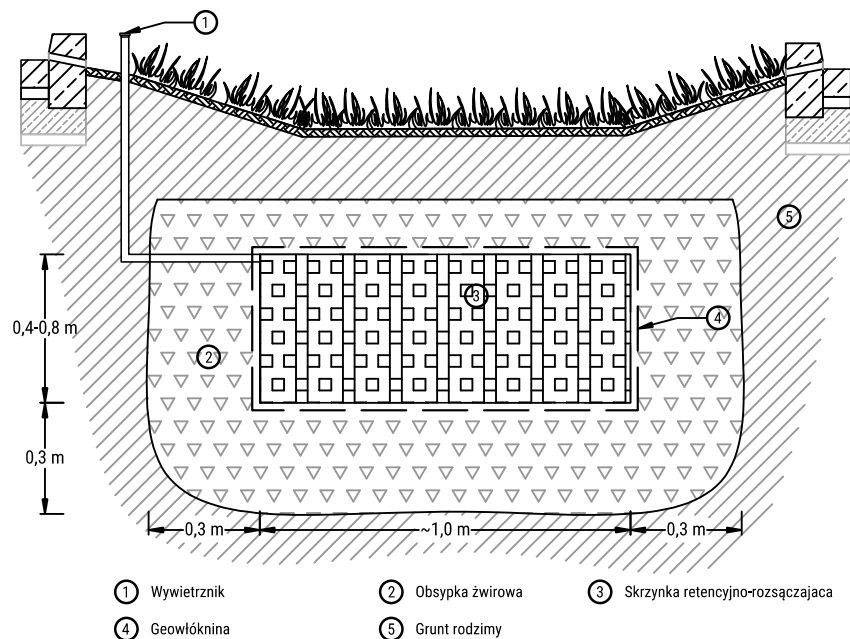
Przykład wykorzystania skrzynek retencyjno-rozsączających w muldzie chłonnej
